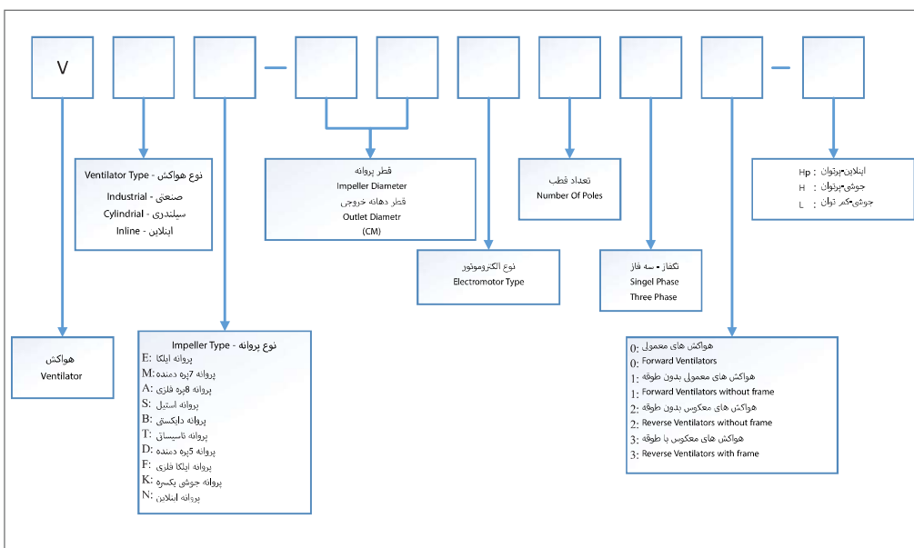
دستورالعمل کدینگ هواکش صنعتی
