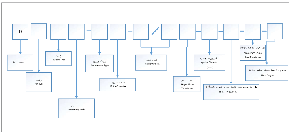
دستورالعمل کدینگ هواکش صنعتی DVMP
