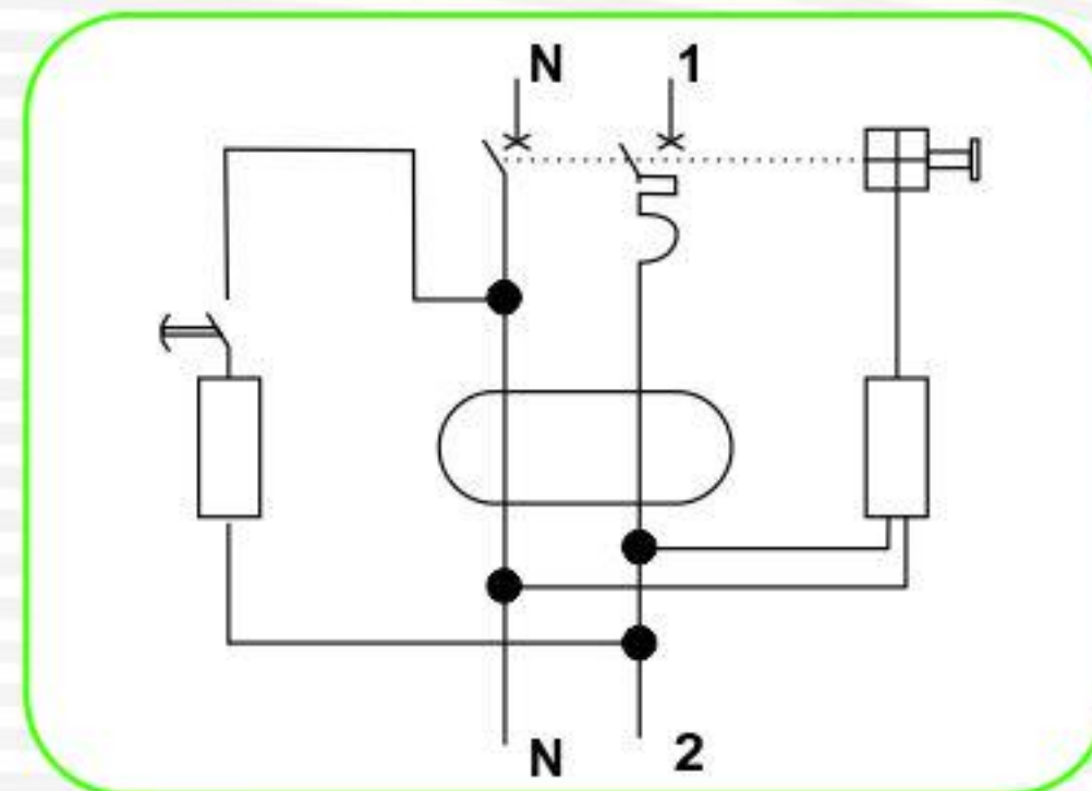
مدار الکتریکی کلید محافظ جان ترکیبی مگنتیک
