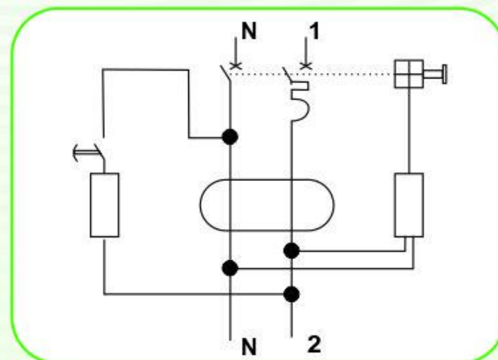
مدار الکتریکی محافظ جان ترکیبی الکترونیکی
