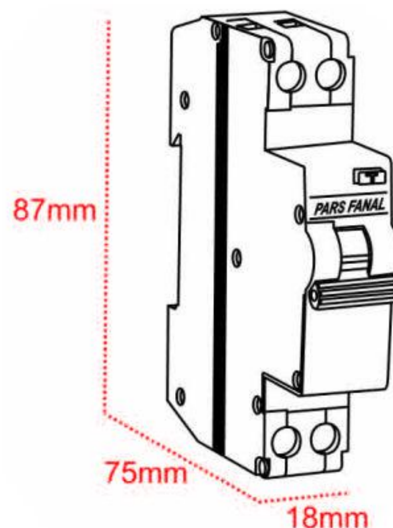
ابعاد و اندازه های مولتی محافظ پارس فانال مدل 25 و 32 PFL
