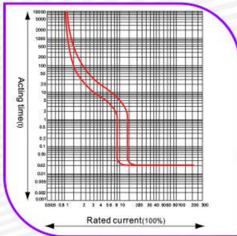
منحنی قطع کلیدهای 250A-FIX
