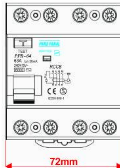
ابعاد و اندازه کلید محافظ جان مدل PFR
